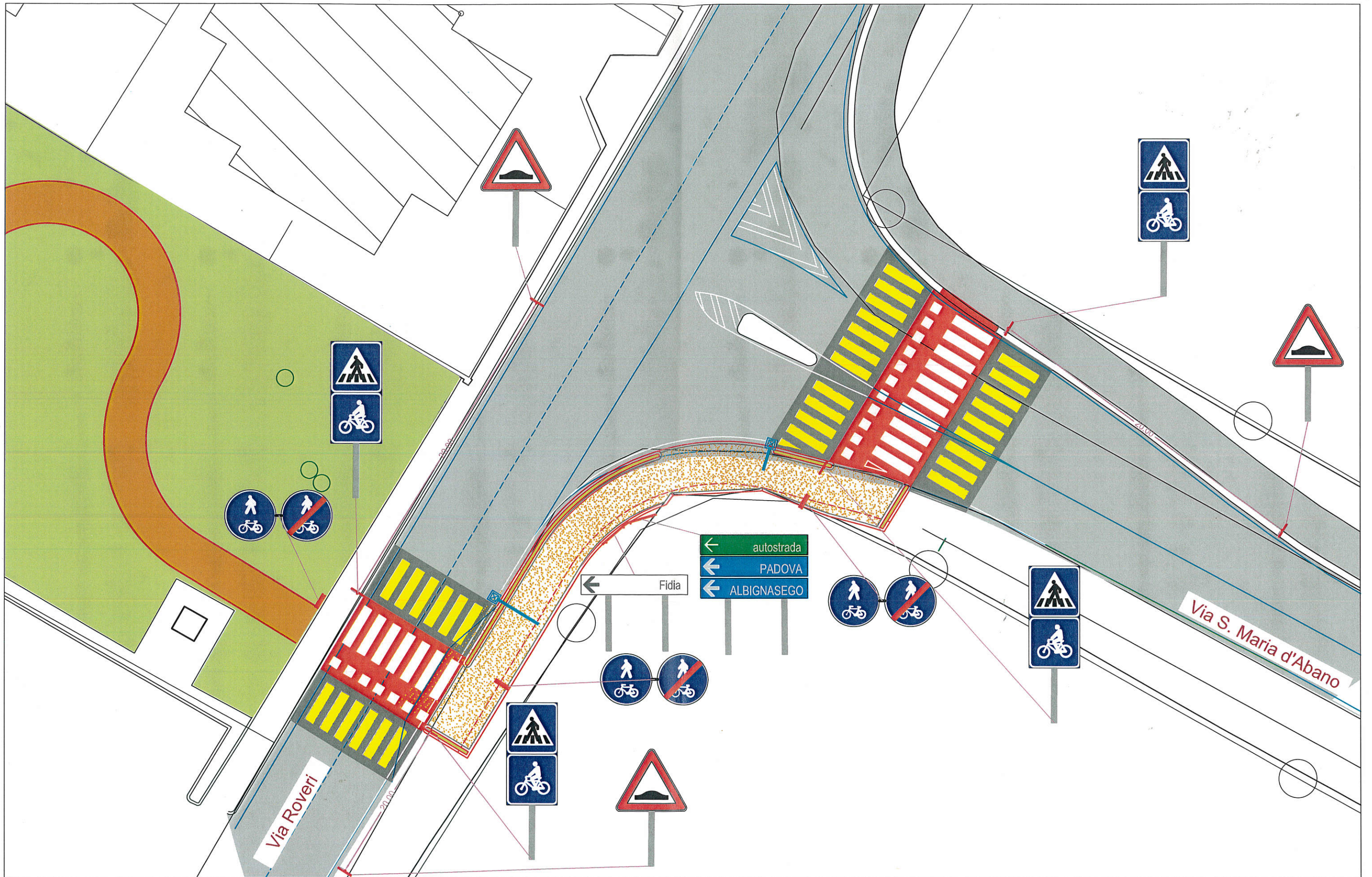
Segnaletica verticale - Località Giarre: incrocio tra Via Roveri e Via S. Maria d'Abano e Parco pubblico Scala 1:200
