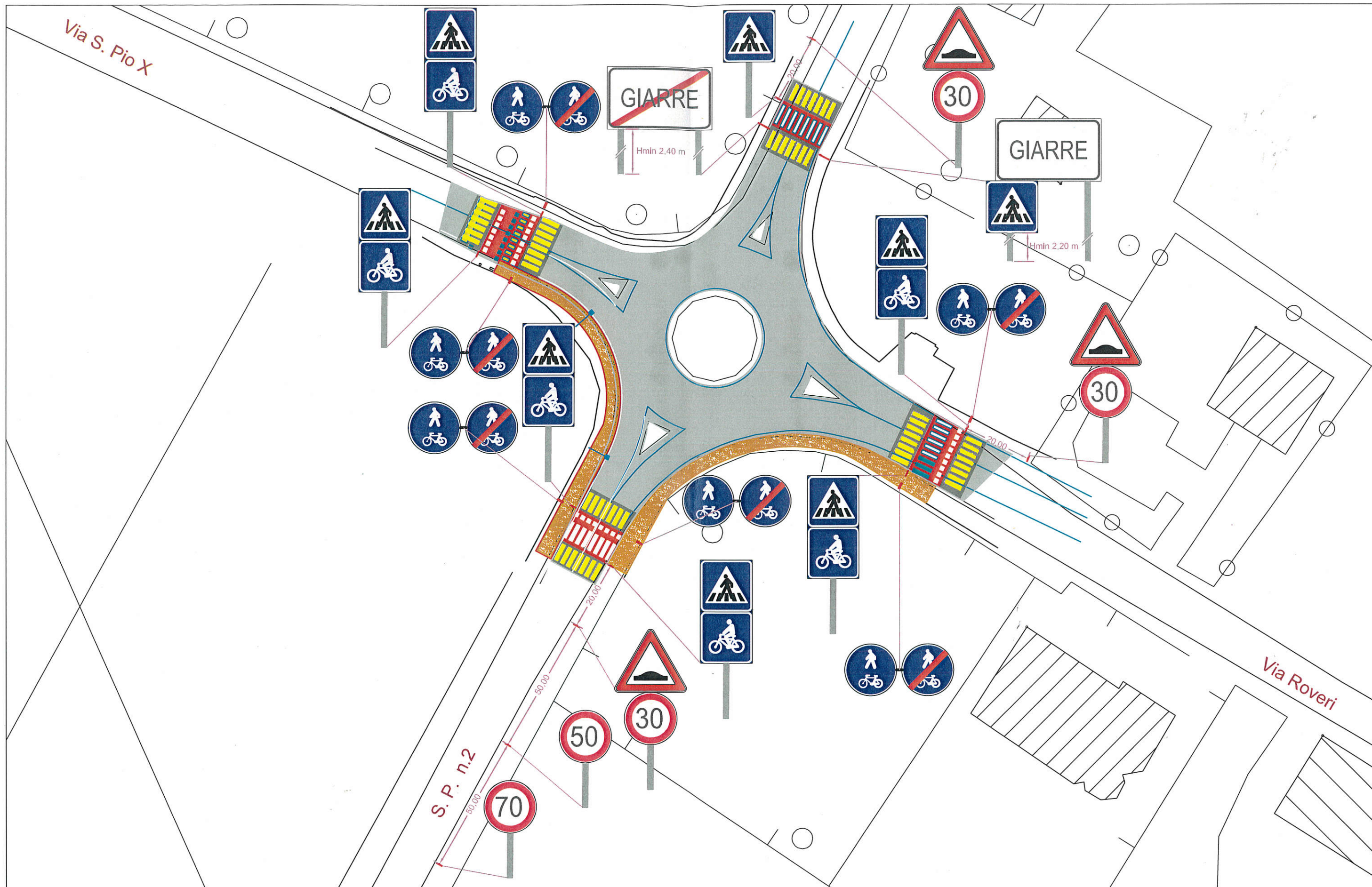
Segnaletica verticale - Incrocio tra S.P. 2 e le Vie S. Pio X e Roveri Scala 1:500
